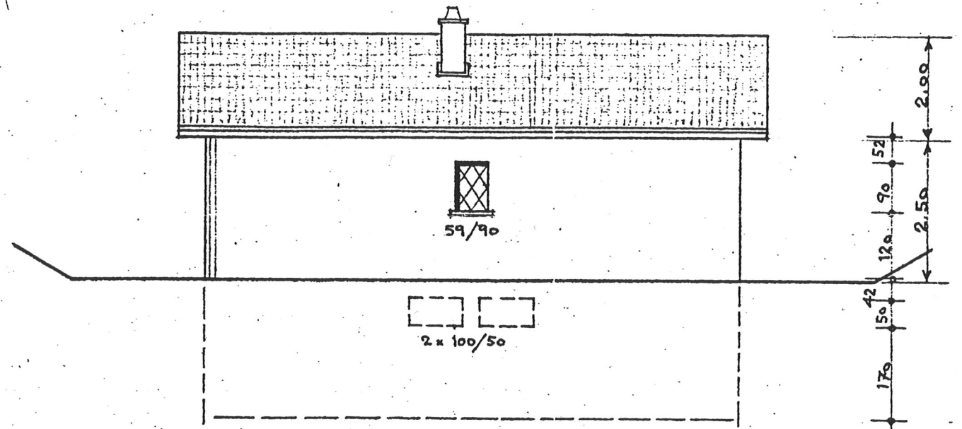
FACADE NORD-OUEST
