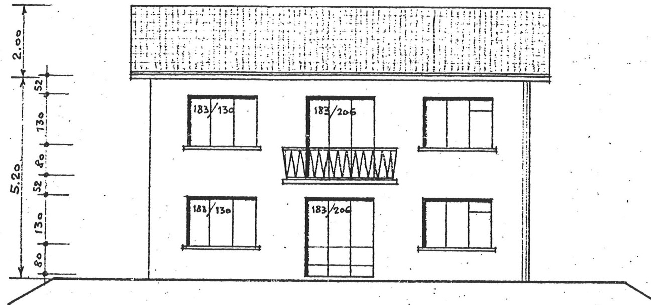
FACADE SUD-EST
