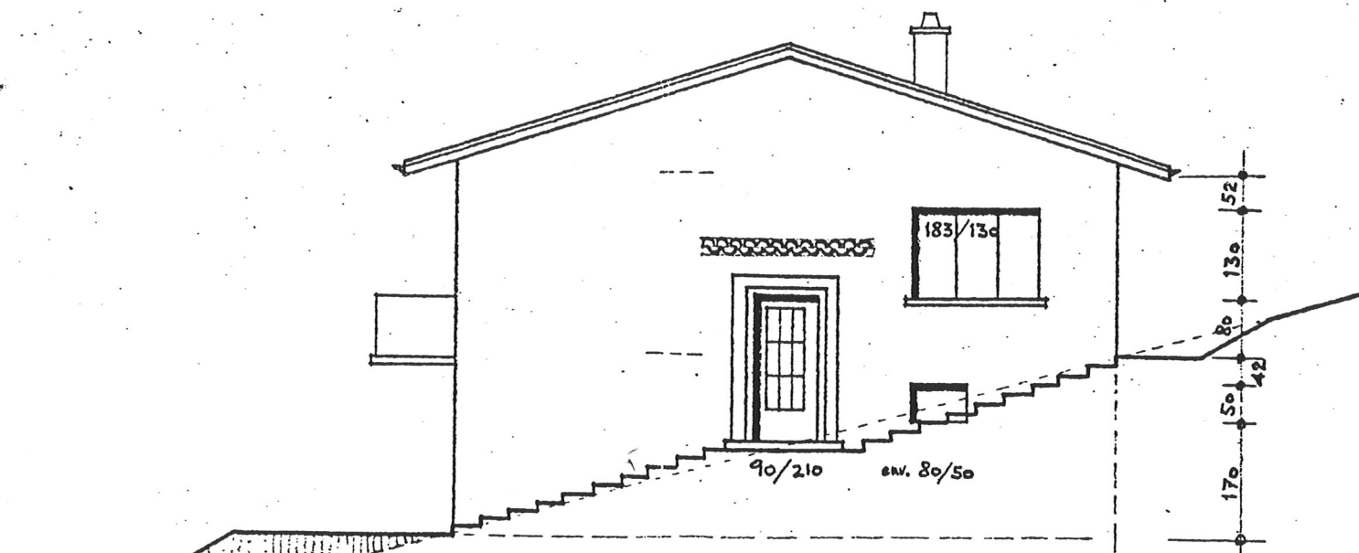
FACADE NORD-EST
